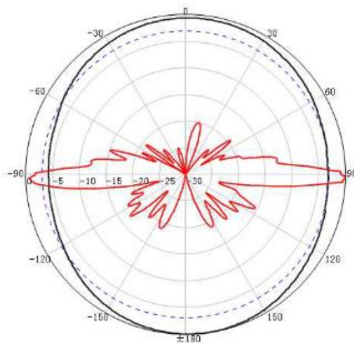
H-Pol @ 2450MHz
